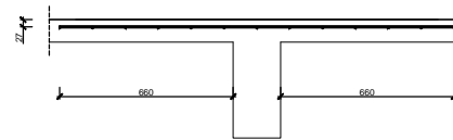
Podciąg skala 1:10
