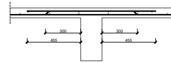
Żebro skala 1:10
